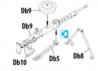
DT 7.62 mm Tank Machine Gun 7,62-мм танковый пулемет Дегтярева ДТ
