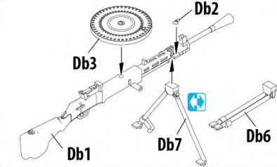
1 DP 7.62 mm Light Machine Gun 7,62-мм ручной пулемет Дегтярева ДП
